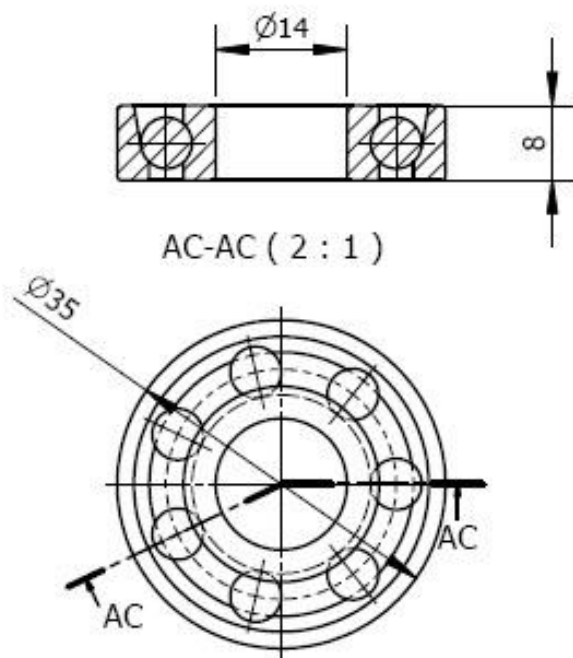
BALL BEARING JIS B 1538 EN 14 14x35x8
