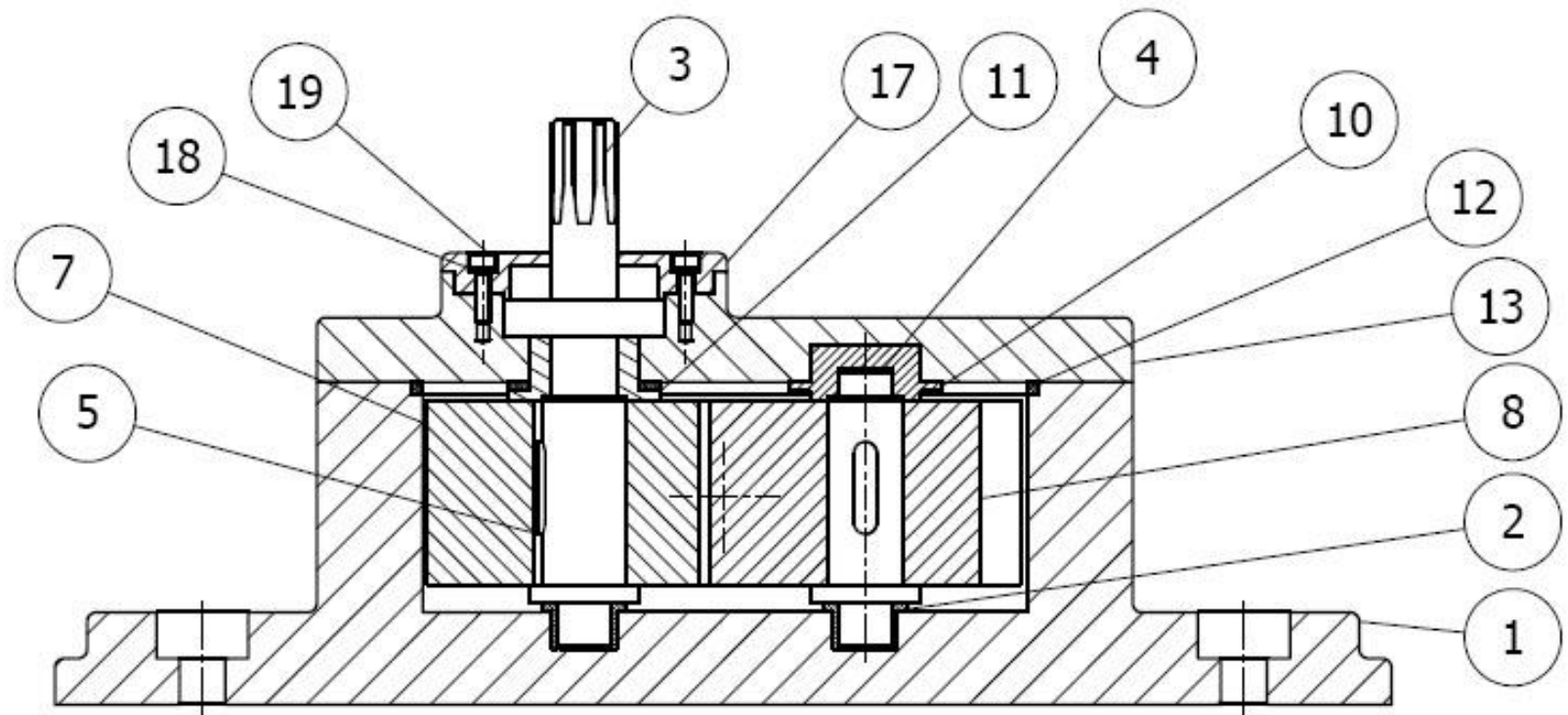
A-A (1:1)
